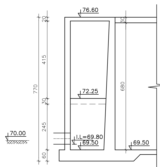
H-H חתך ק"נ 1:100
