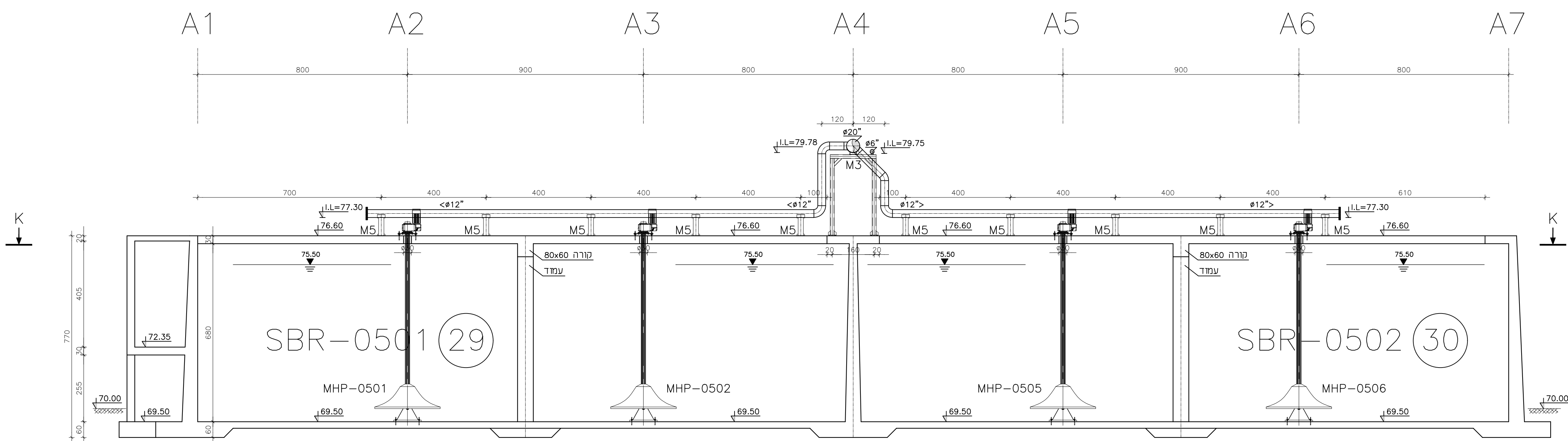
G-G חתך ק"נ 1:100
