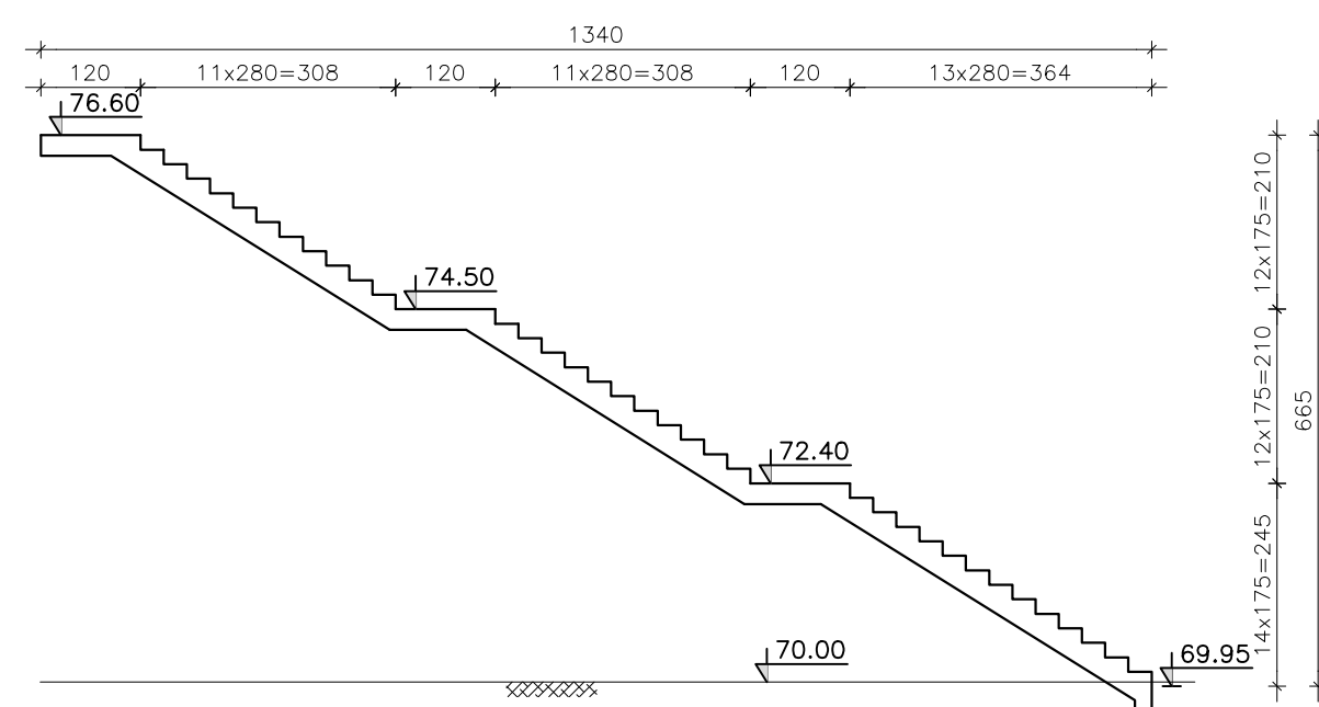
T-T חתך ק"נ 1:100
