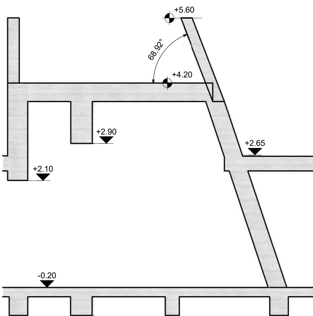
4-4 1 : 50
