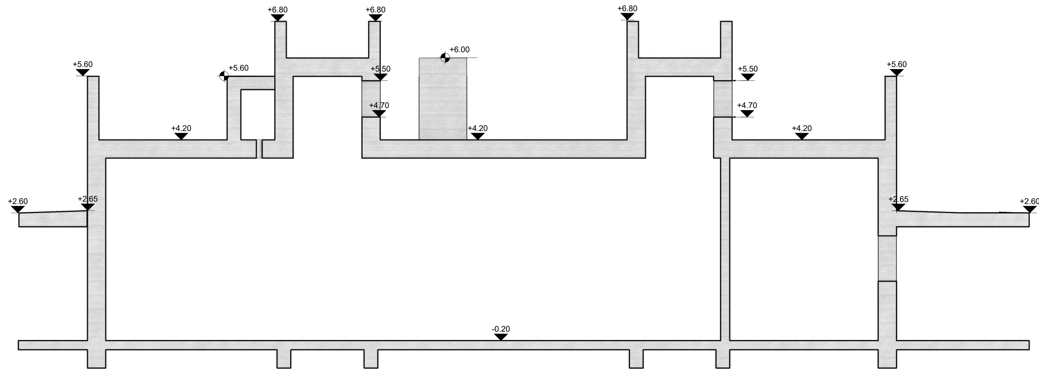
2-2 1 : 50
