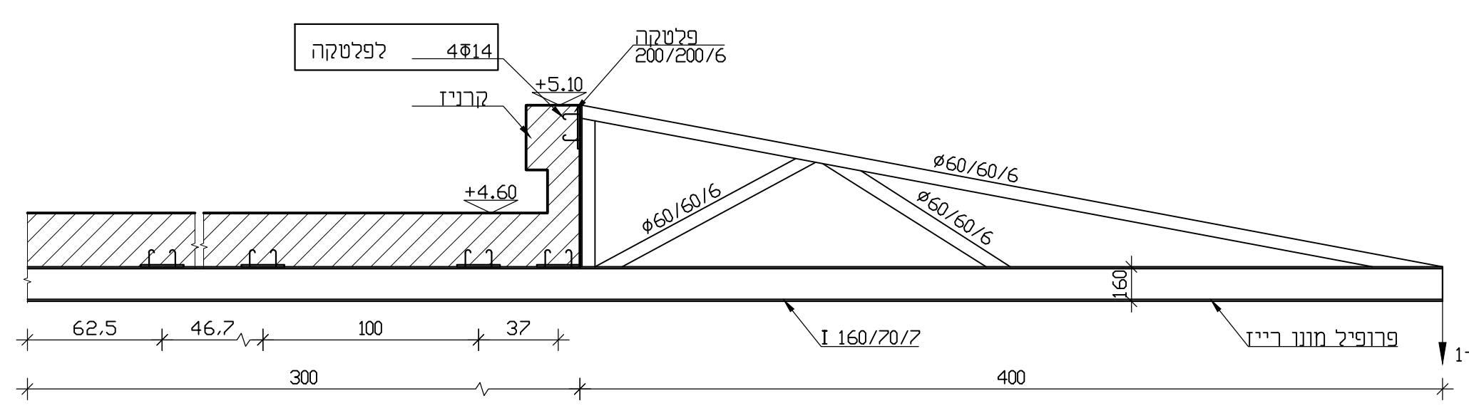
פרט חיבור פרופיל ל גג בשון 1:25
