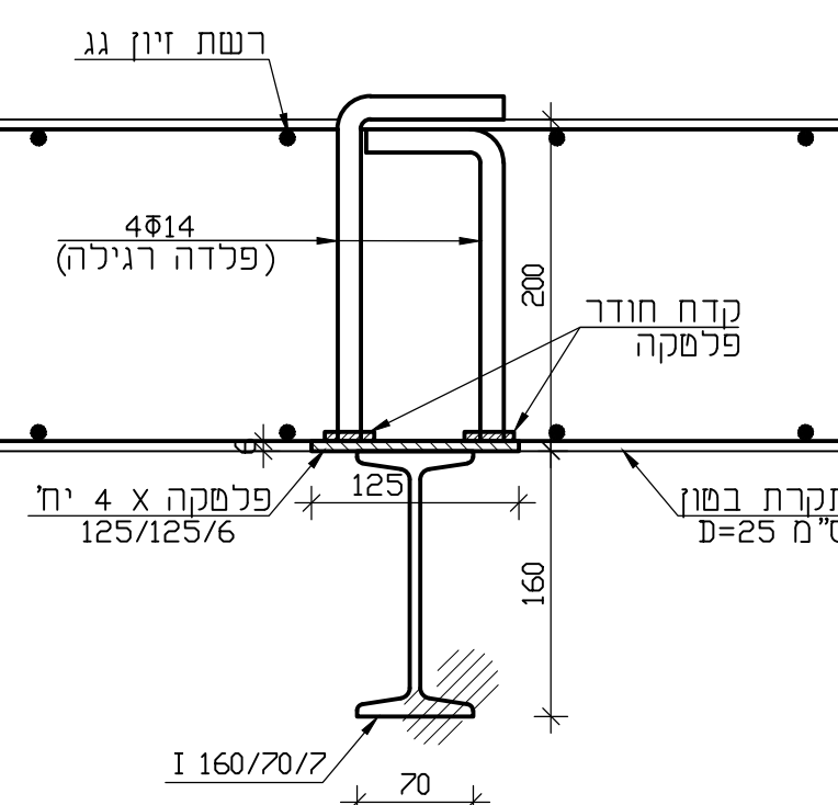
פרט חיבור פרופיל ל גג בשון 1:5
