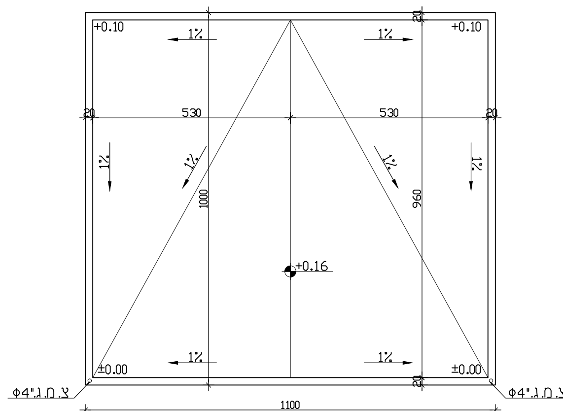
תכנית שיפועי ניקוז גג בשון 1:100
