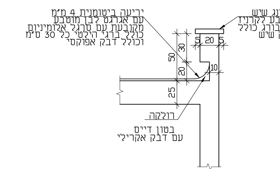
חור 1-1 פרט איטום קרניז 1:25
