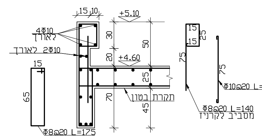
חור ב-ב 1:25
